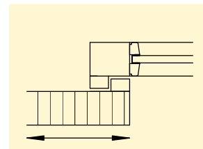
Verglasung Standard Schiebetür Vollbau
