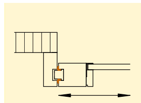
Seitenteil Vollbau Schiebetür Vergl. eins. bündig
