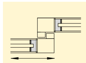
Verglasung PLANLINE Schiebetür PLANLINE
